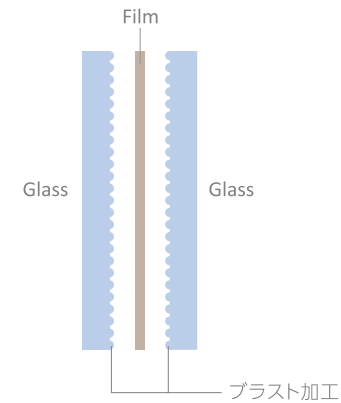
<インナーブラストガラスの構造>
